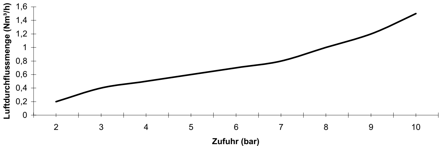
DIAGRAMM LUFTKONSUM
